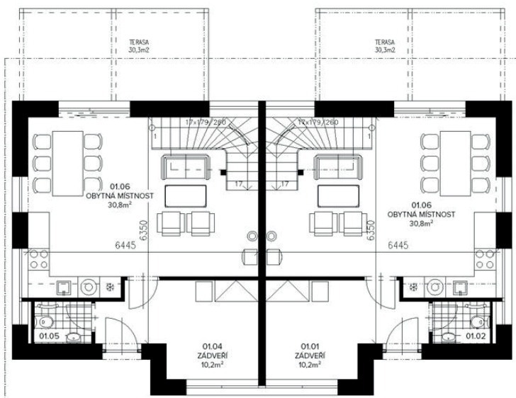
PŮDORYS 1.NP
