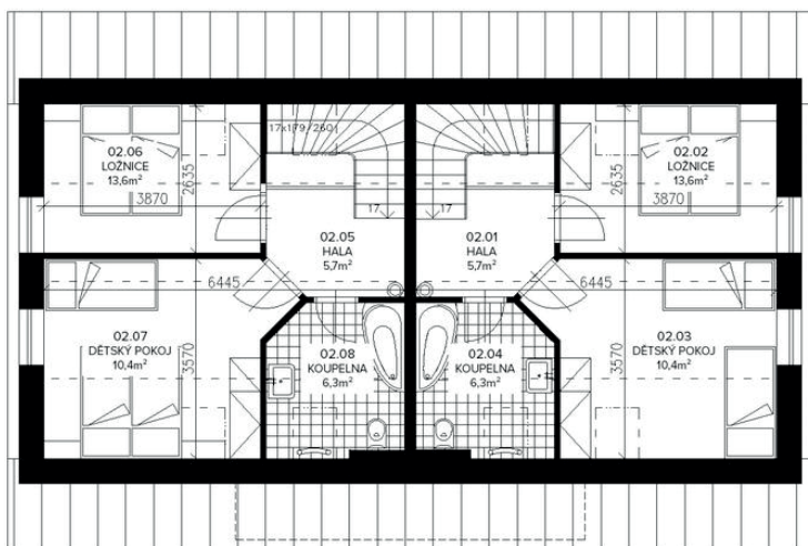
PŮDORYS 2.NP
